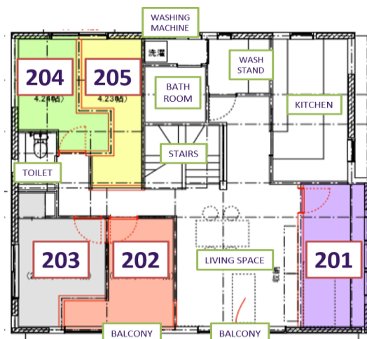
2F
